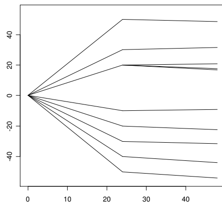
Figura 4.5: Arbre reduït 10 escenaris
