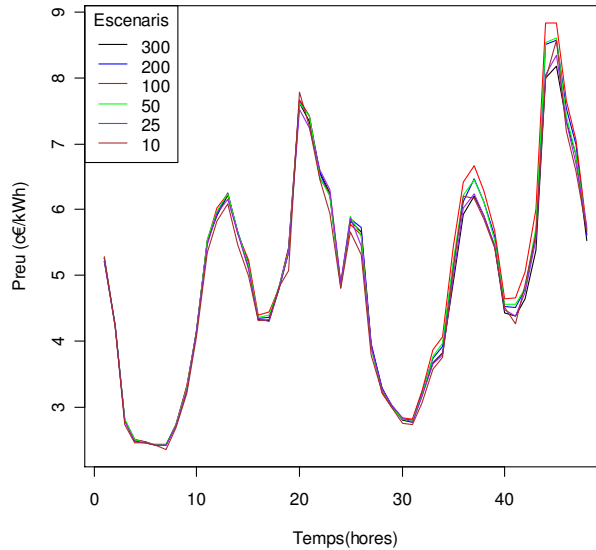
Figura 4.12: Comparació mitjanes horàries arbre escenaris reduïts
