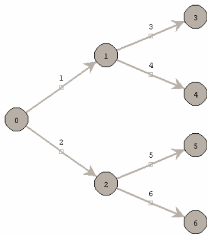
Figura 3.2: Exemple d'arbre d'escenaris
