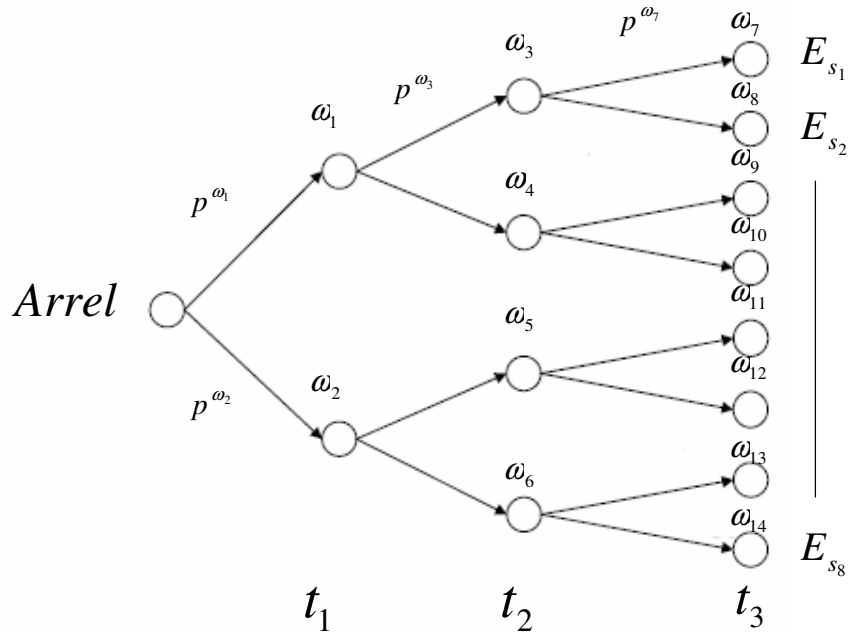
Figura 2.7: Arbre d'escenaris amb bifurcacions a cada node
