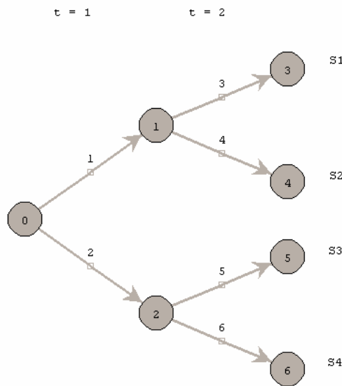
Figura 3.3: Exemple d'arbre d'escenaris amb etapes i escenaris
