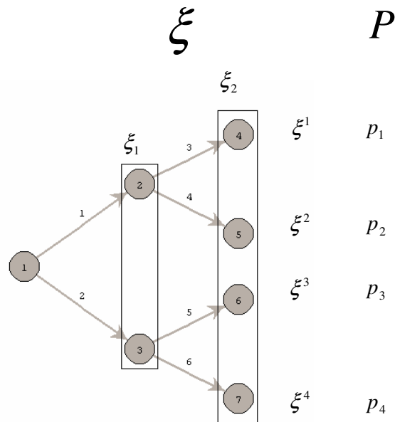
Figura 3.1: Representació d'un arbre d'escenaris de dues etapes
