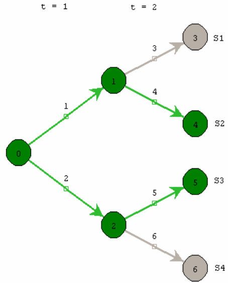
Figura 3.6: Arbre d'escenaris reduït
