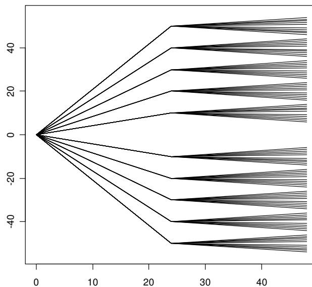
Figura 4.1: Representació Arbre 100 escenaris
