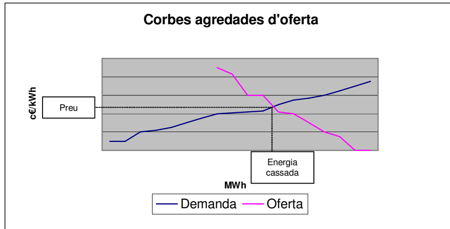
Figura 2.2: Corbes agregades d'oferta
