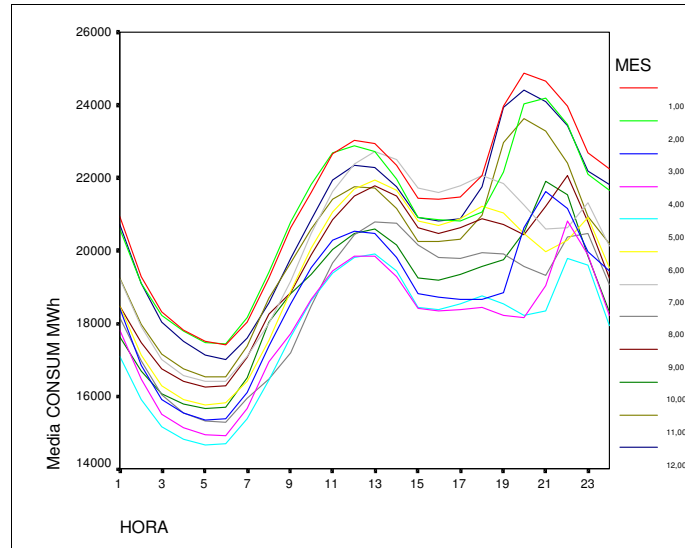
Figura 2.5: Corba consum mitjà horari pels diferents mesos
