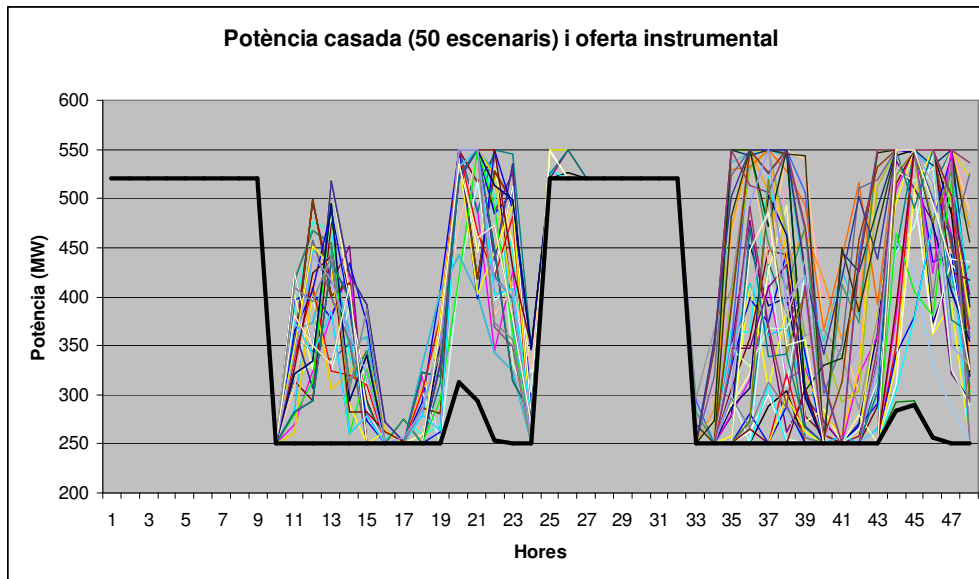
Figura 4.15: Potència cassada per 50 escenaris i oferta instrumental tèrmica 2
