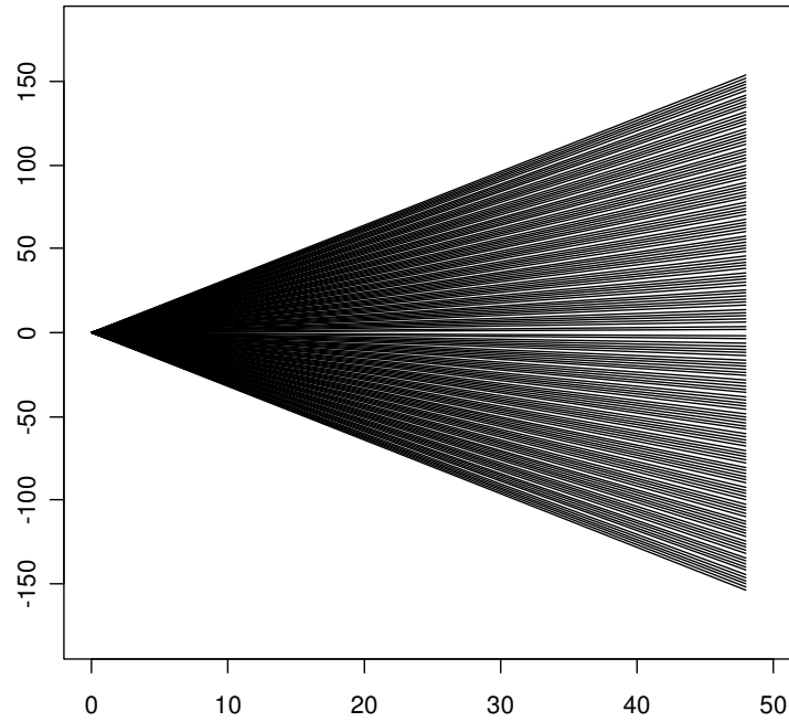
Figura 4.6: Fan de 154 escenaris
