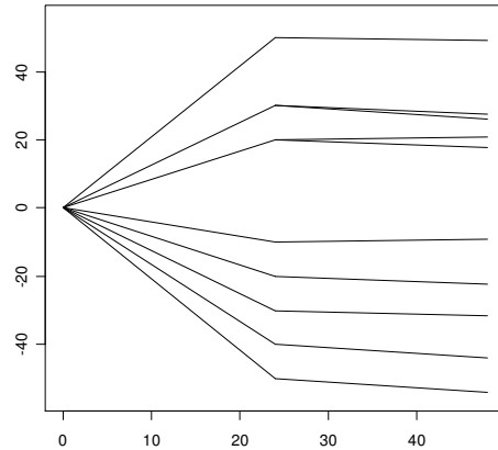
Figura 4.3: Arbre reduït 10 escenaris
