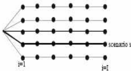
Figura 2.8: Arbre d'escenaris tipus fan
