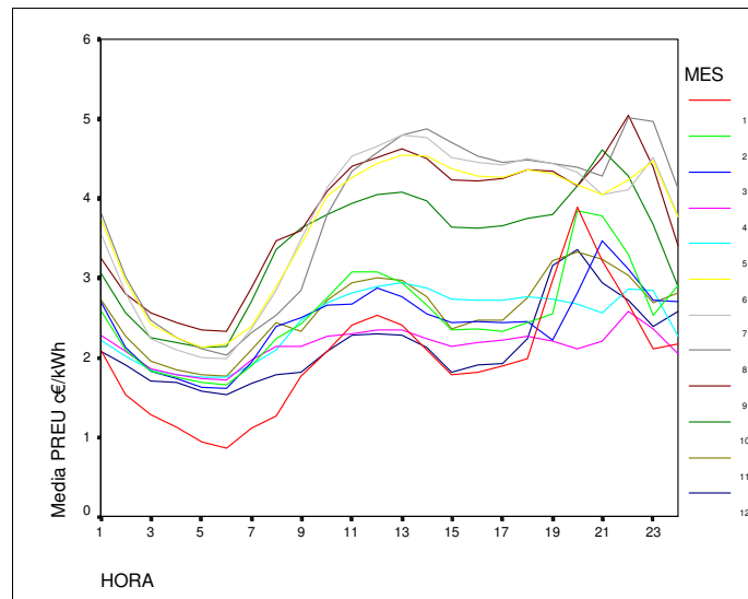
Figura 2.6: Corba mitjana preu horari pels diferents mesos
