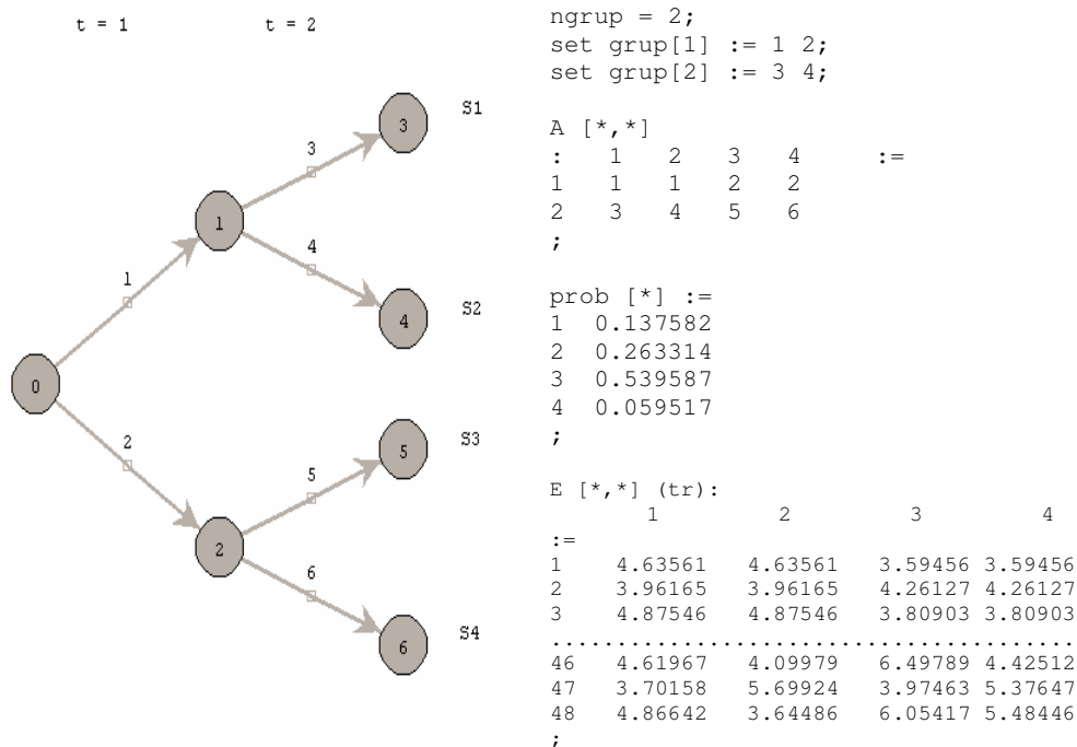
Figura 3.5: Arbre d'escenaris inicial
