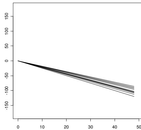
Figura 4.8: Fan reduït 10 escenaris
