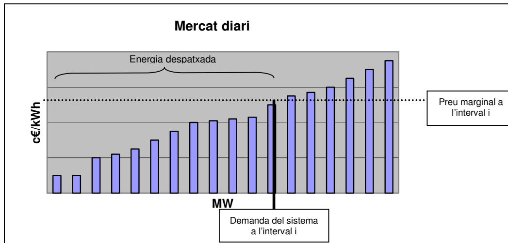
Figura 2.1: Ofertes presentades pels grups generadors
