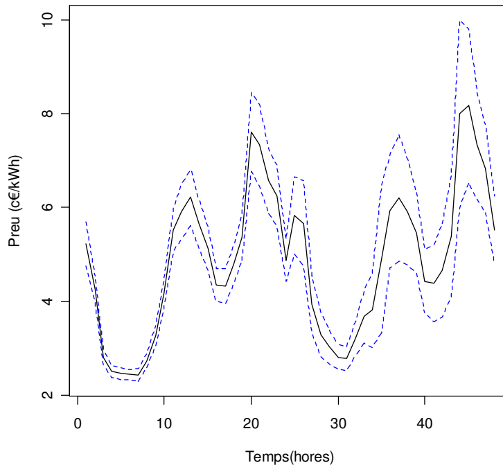
Figura 4.11: Mitjanes més desv. estàndards horàries arbre 300 escenaris
