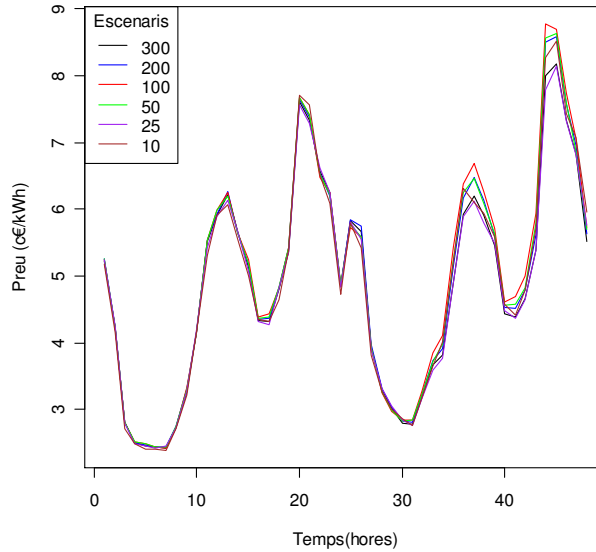
Figura 4.13: Comparació mitjanes horàries arbre escenaris reduïts
